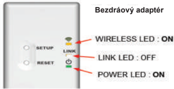
Bezdrátový adaptér
